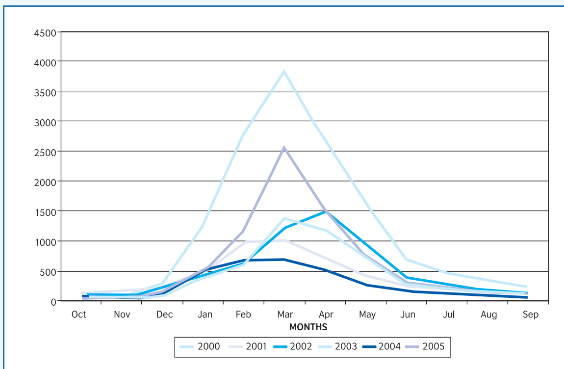
Figure 4.3: Hydrograph for Kafue Hook Bridge
